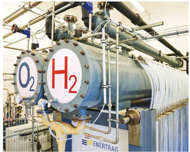
In Prenzlau (Brandenburg) ist seit 2011 das weltweit erste Wasserstoff-Hybridkraftwerk in Betrieb.
